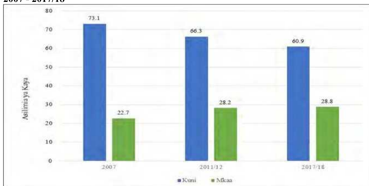
Kielelezo Na. 20.8: Mwenendo wa Matumizi wa Nishati ya Kuni na Mkaa Mwaka 2007 - 2017/18
